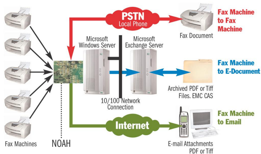
Microsoft Exchange Server 2003 與 NOAH 整合架構圖
